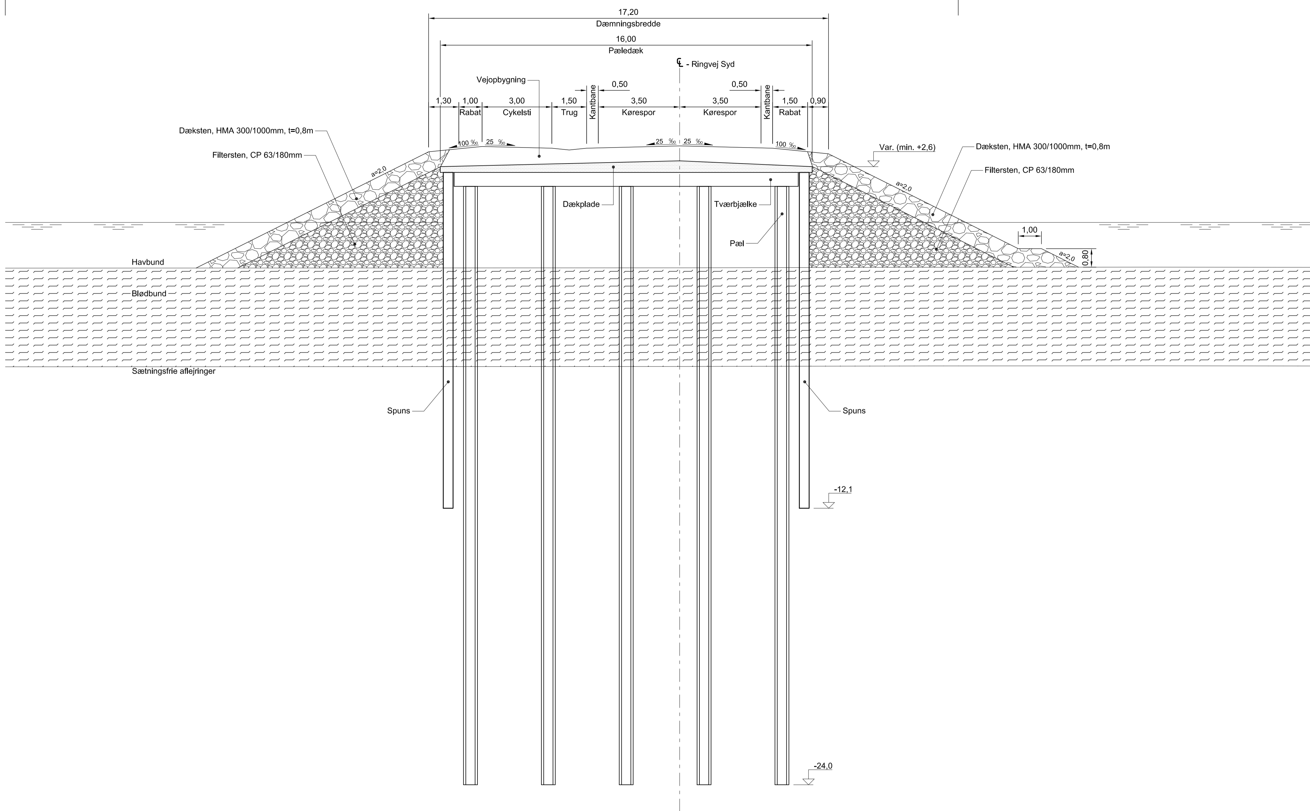
SNIT B-B, 1:100 Tværsnit i Ringvej Syd i dæmning ved Bygholm A.
