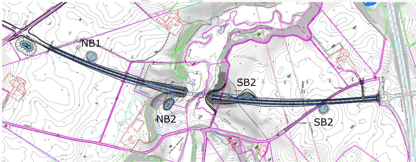
Figur 1: Ny forbindelsesvej og regnvandsbassiner.
