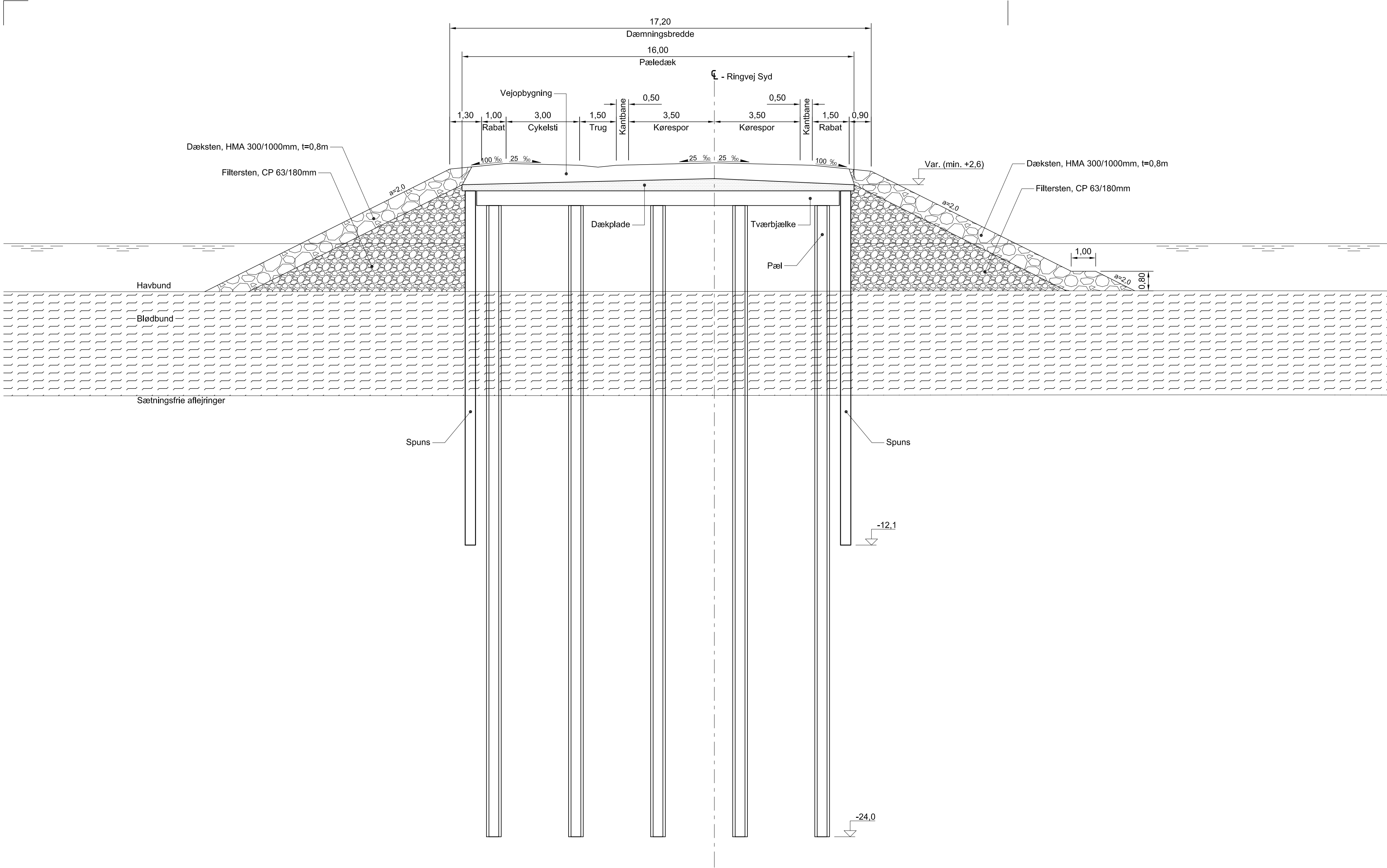
SNIT B-B, 1:100 Tværsnit i Ringvej Syd i dæmning ved Bygholm A.
