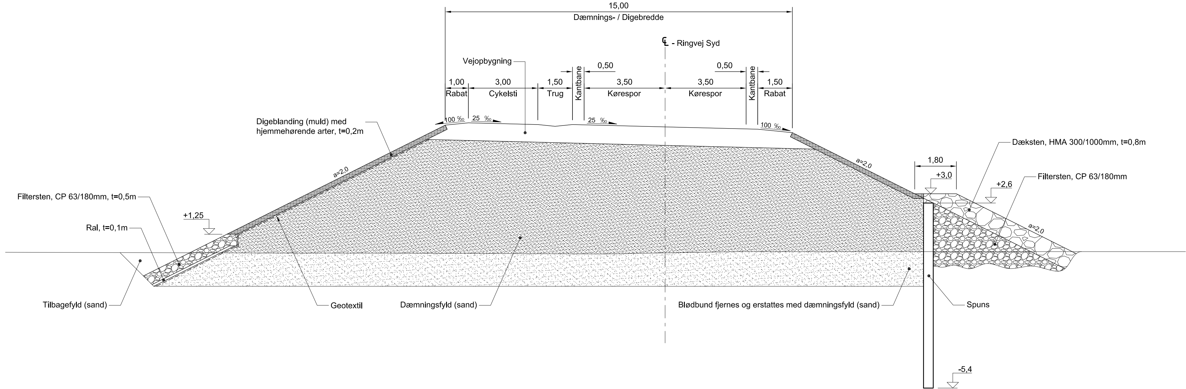
SNIT A-A, 1:100 Tværsnit i Ringvej Syd i dæmning ved Dagnæs Bæk.
